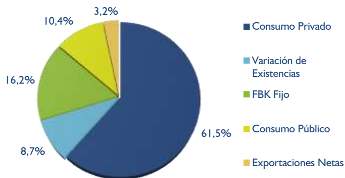
Estructura - Demanda
