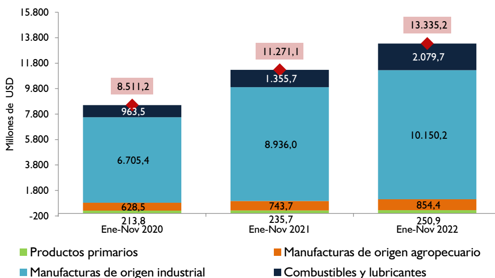
Gráfico 18 Evolución de las importaciones por niveles de procesamiento en millones de dólares FOB Enero – Noviembre 2020 / Enero – Noviembre 2022
