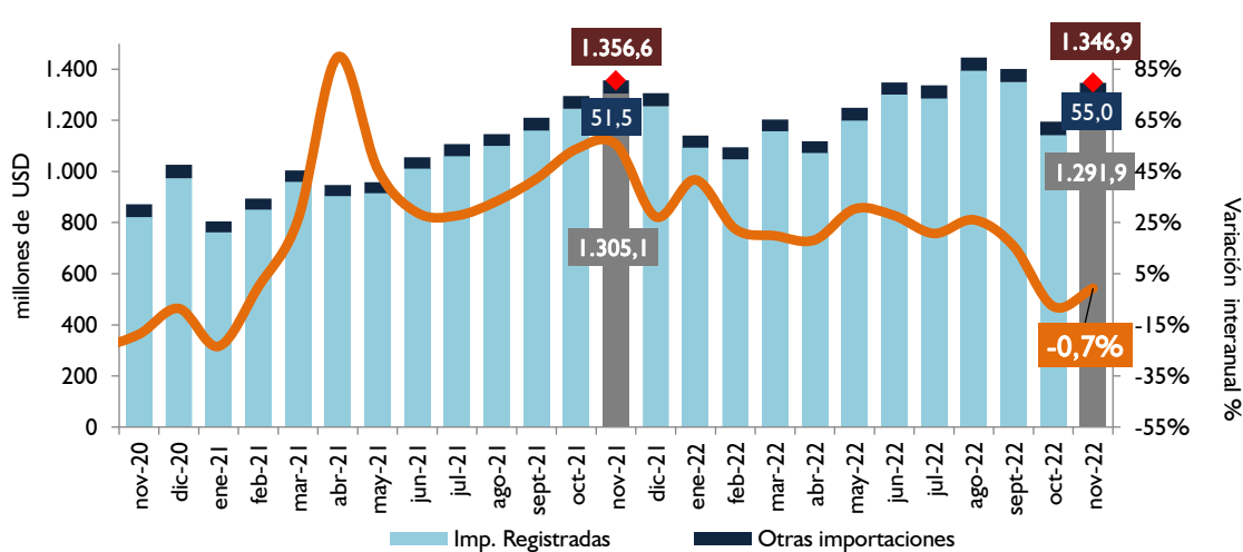
Gráfico 13 Evolución mensual de las importaciones totales Noviembre 2020 / Noviembre 2022
