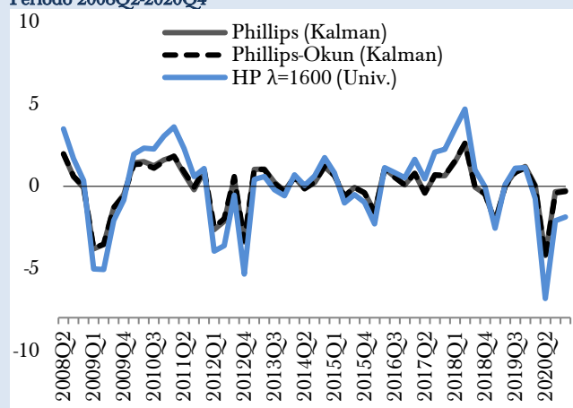
Gráfico 1 Evolución de la Brecha del Producto Periodo 2008Q2-2020Q4
